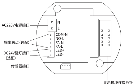
图 4-2 接线示意图
