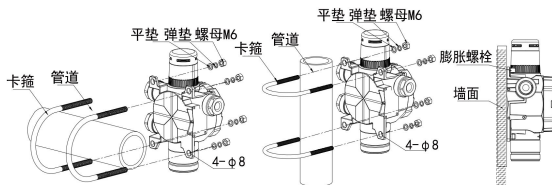
图 4-1 安装示意图
