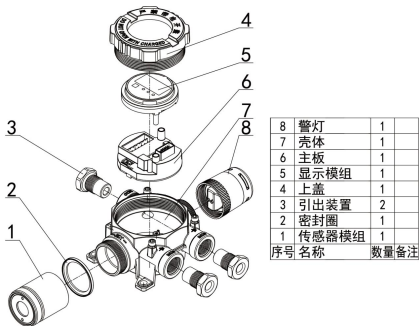
图 2-2 组成结构示意图
