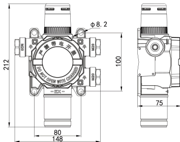
图 2-1 外形尺寸示意图（单位：mm）
